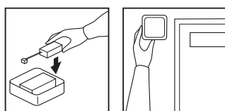
Bluetooth®レシーバーの取付け (取付説明書MAP-801)
